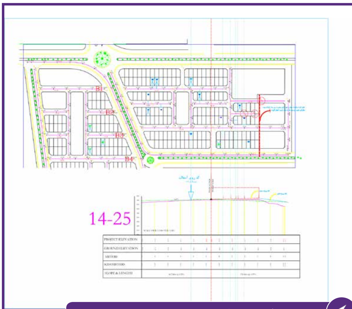
نمونه نقشه پروفیل طولی معابر تهیه شده در واحد نقشه برداری خمینی شهر
